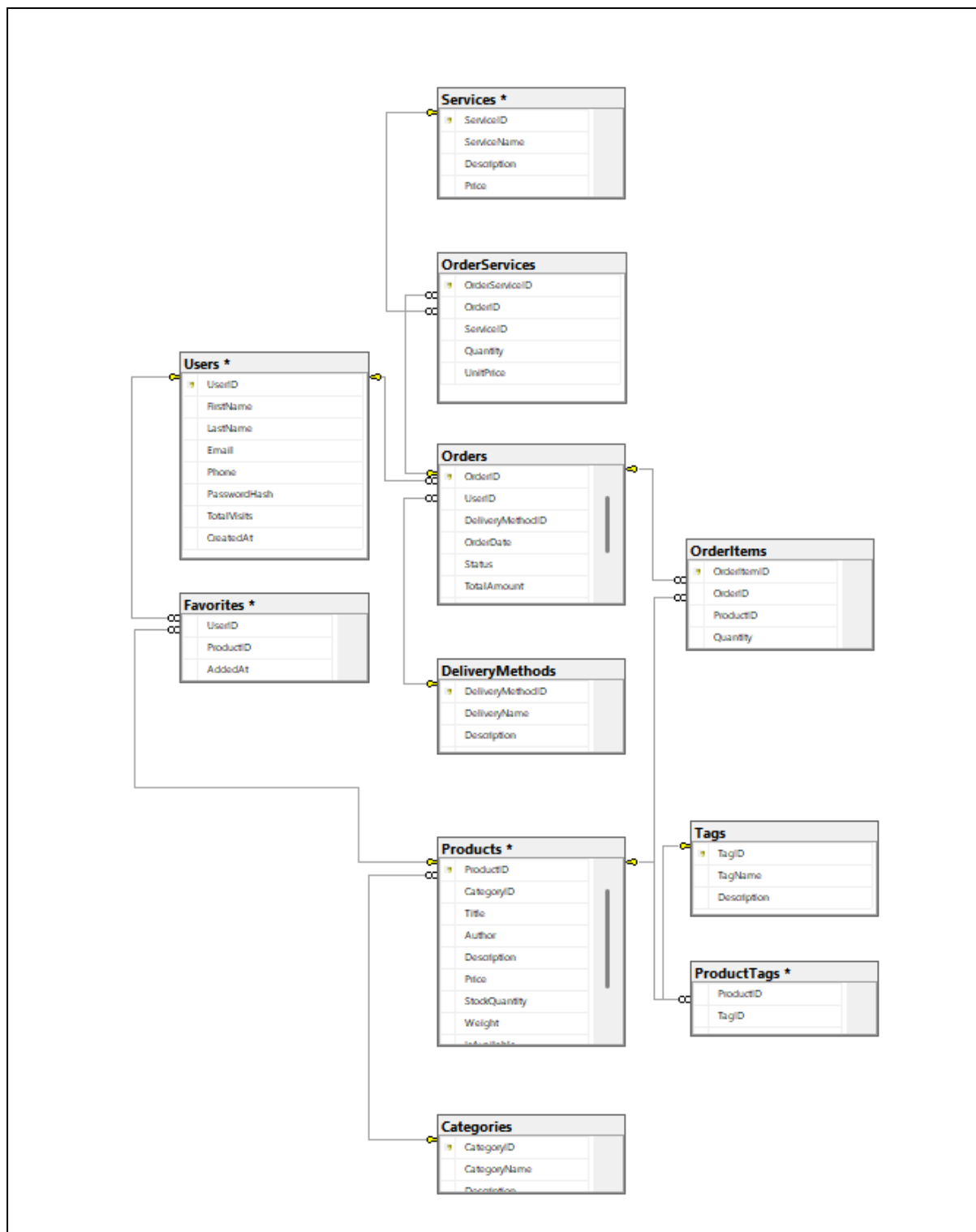
Рисунок 1 – ER-диаграмма базы данных интернет-магазина “В стране книг”
